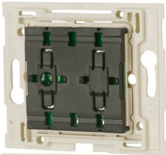
RF Tlačítko 4-bodové - NIKO, baterie 3V
